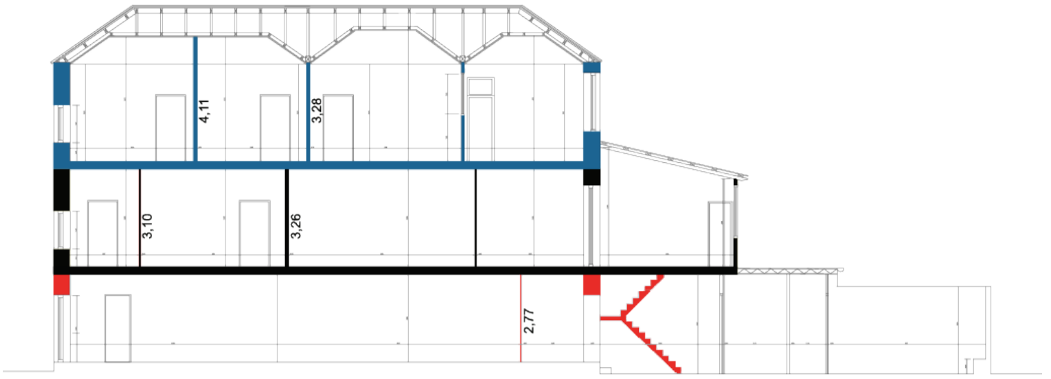
Porta33 - Corte Lateral
